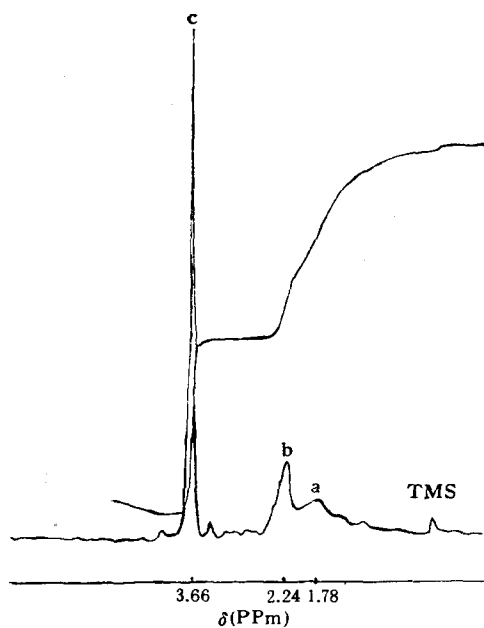
图2 MA 与 MMA 混合投料 GTP 产物 ^1\text{H} -NMR
