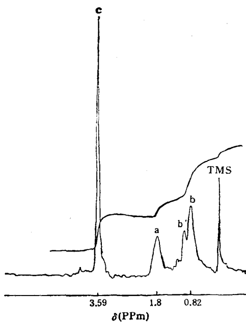
图3 MMA 的 GTP 均聚物 ^1\text{H} -NMR
